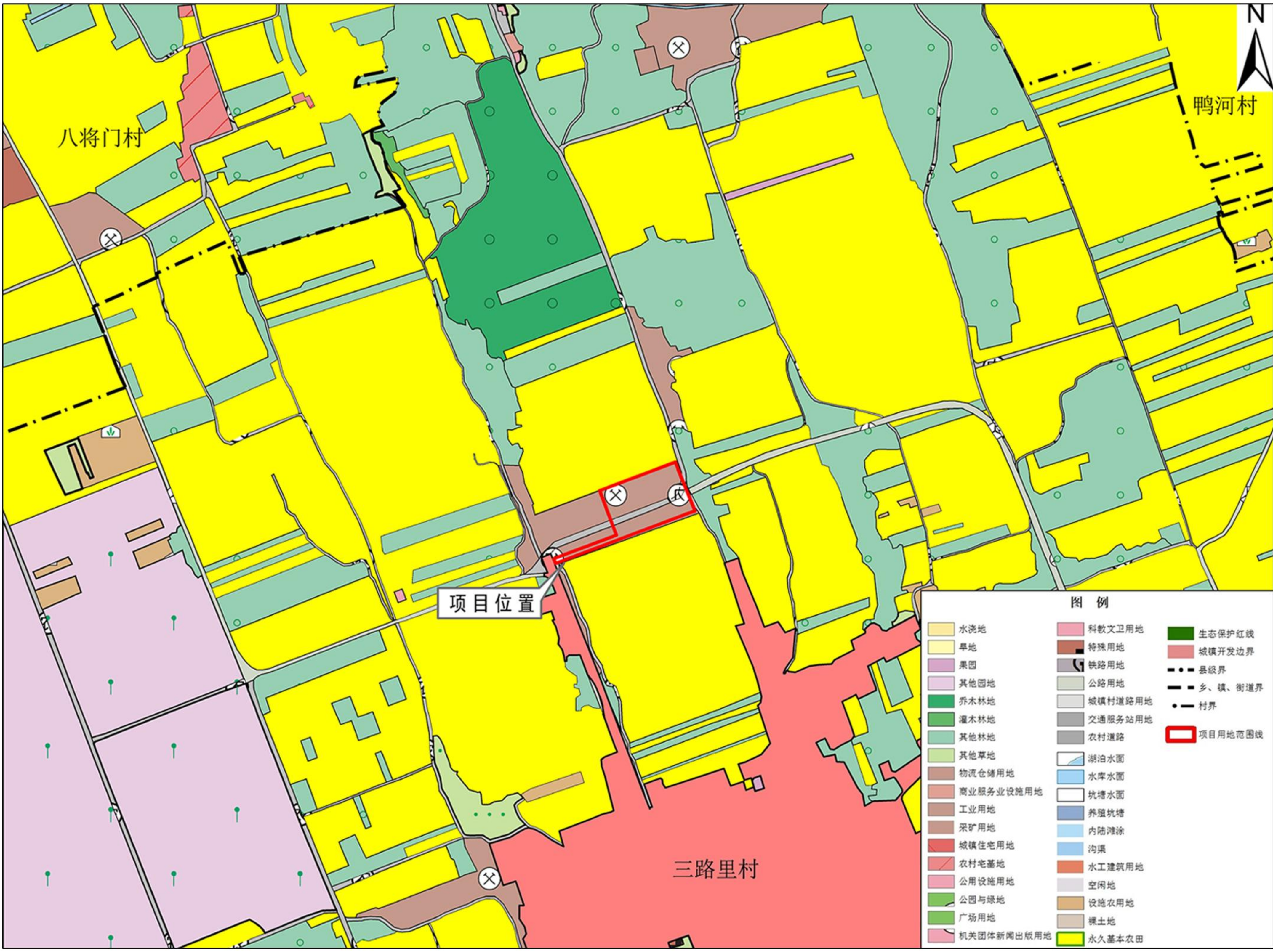
升压站套合“三区三线”划定成果图
