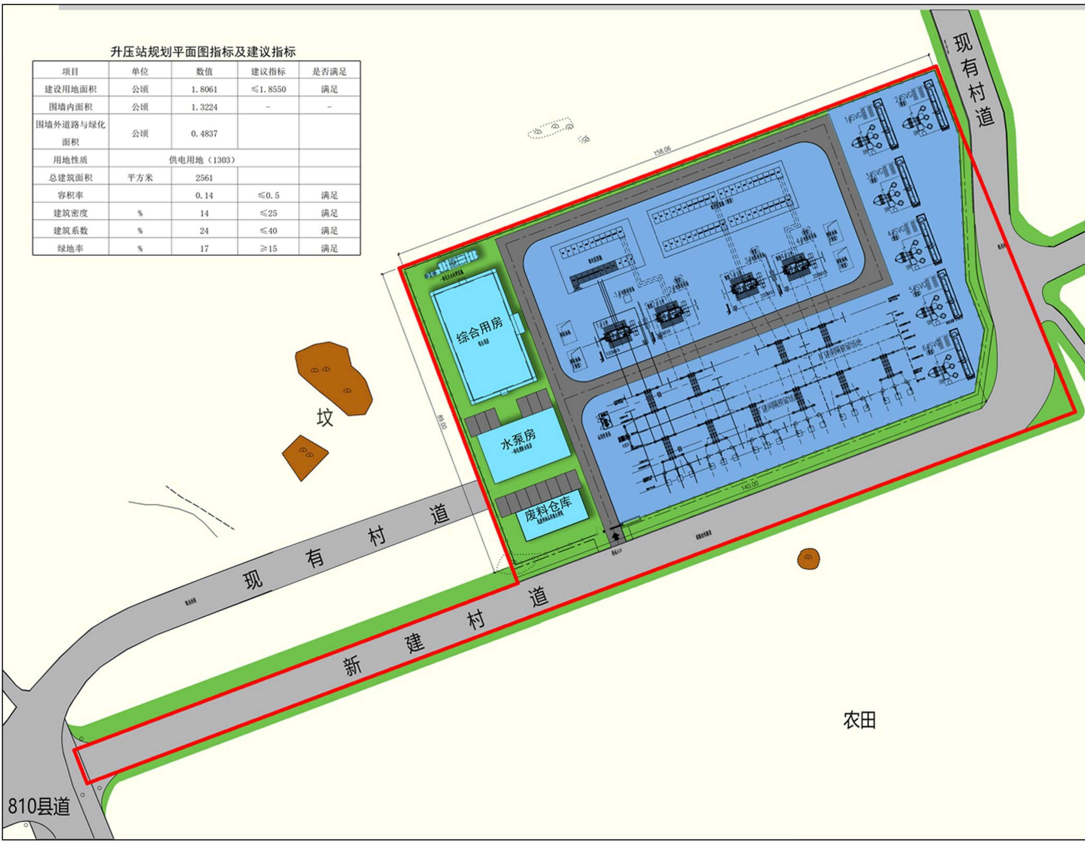
项目总平面布置图
